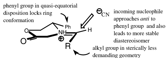
Fig. 2 Stereochemical rationale.
